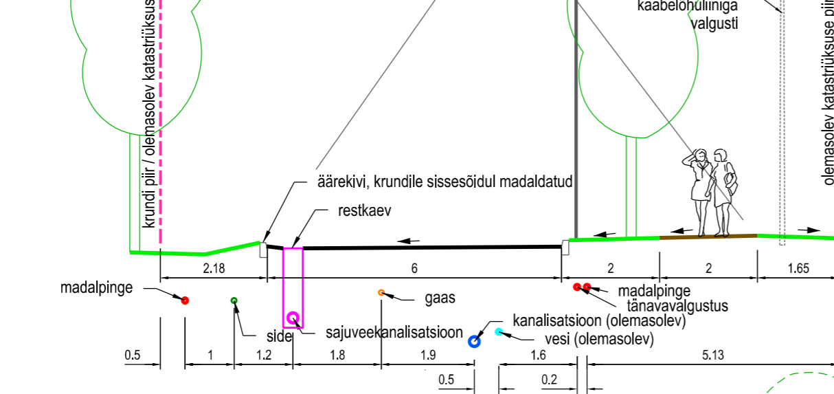
HIPODROOMI TÄNAVA LÕIGE 2-2
