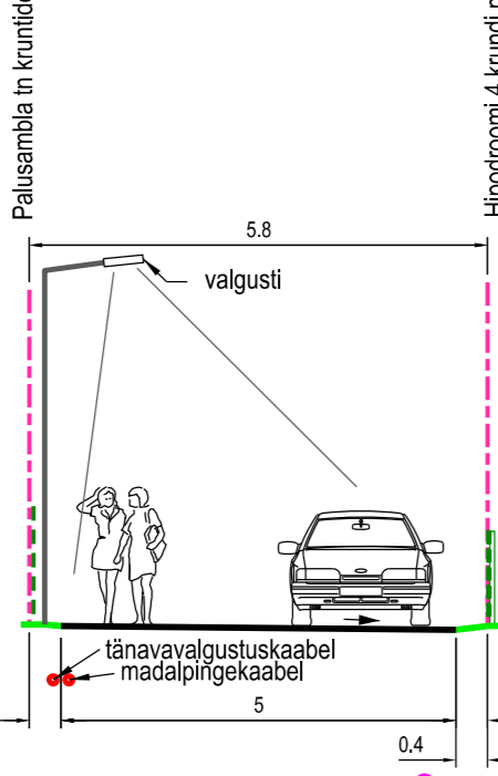
PALUSAMBLA TN KRUNTIDE JA HIPODROOMI 4 KRUNDI VAHELINE TEE LÕIGE 3-3
