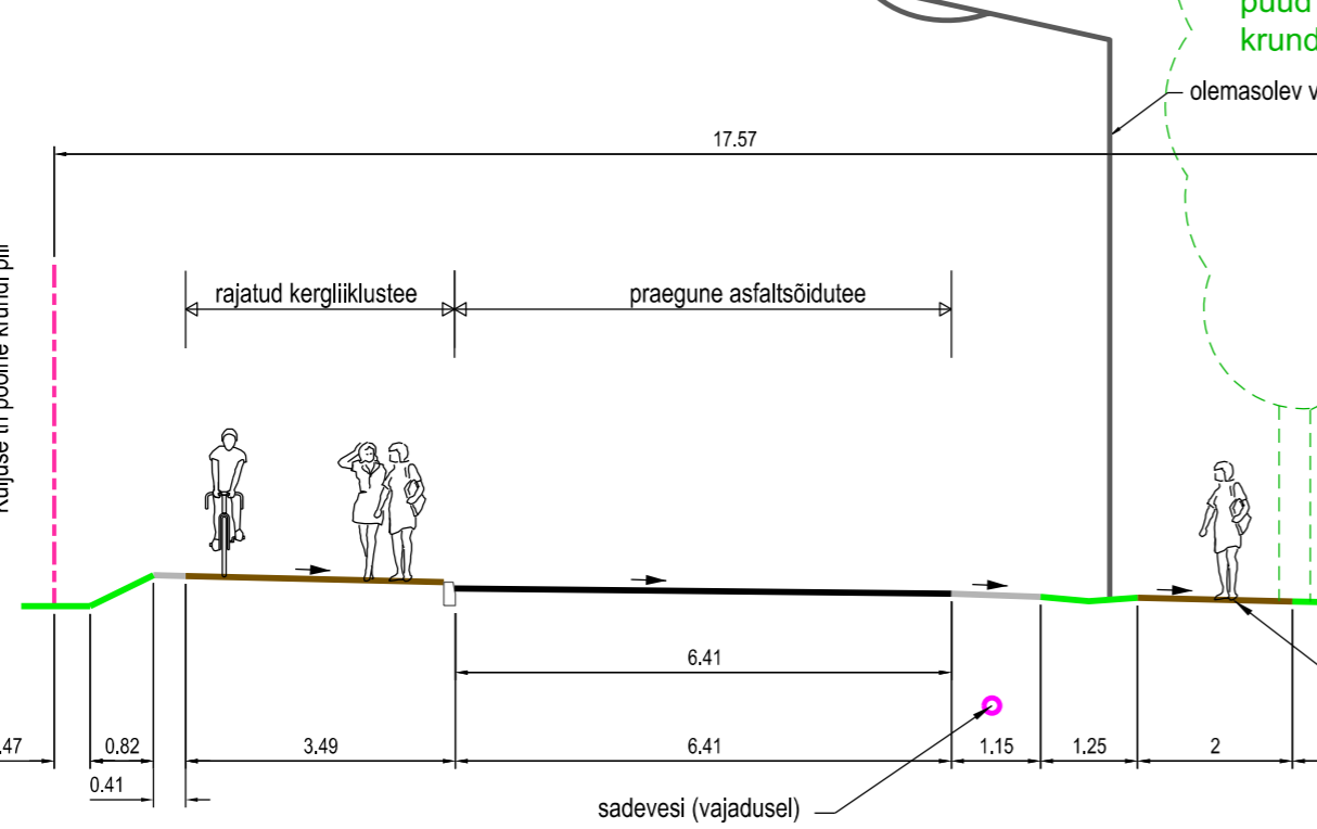
HIPODROOMI TÄNAVA LÕIGE 2-2
