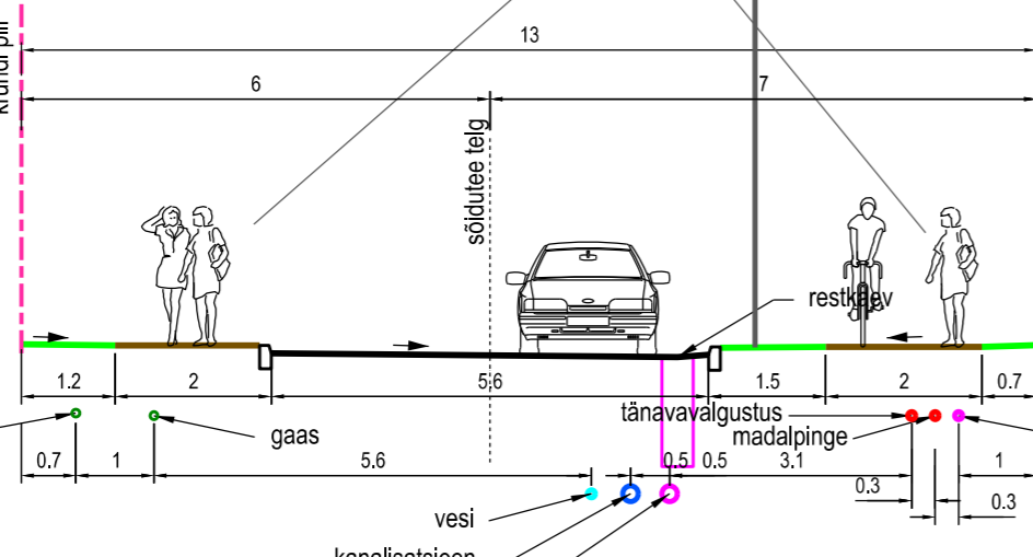
PLANEERITUD TÄNAVA LÕIGE 1-1
